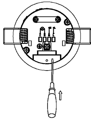
2. Het voorbereiden van de aansluitklem.
