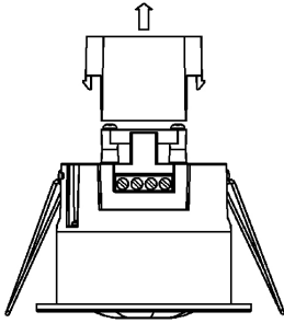
1. Het verwijderen van de vinyl afdekking.
