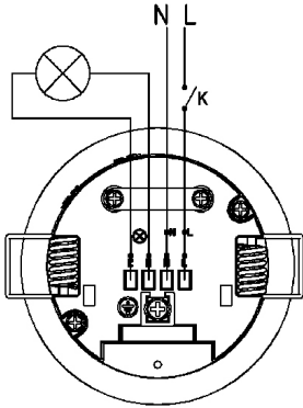
3. Bedrading van de bewegingssensor.
