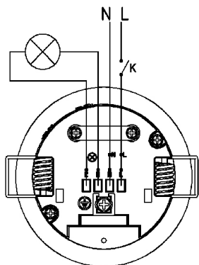
3. Verkabelung des Bewegungssensors.
