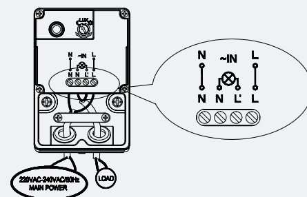
VERDRÄHTUNGSPLAN
